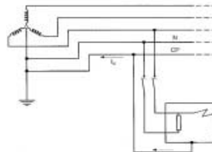
Figura 3. Esquema TN-S.
